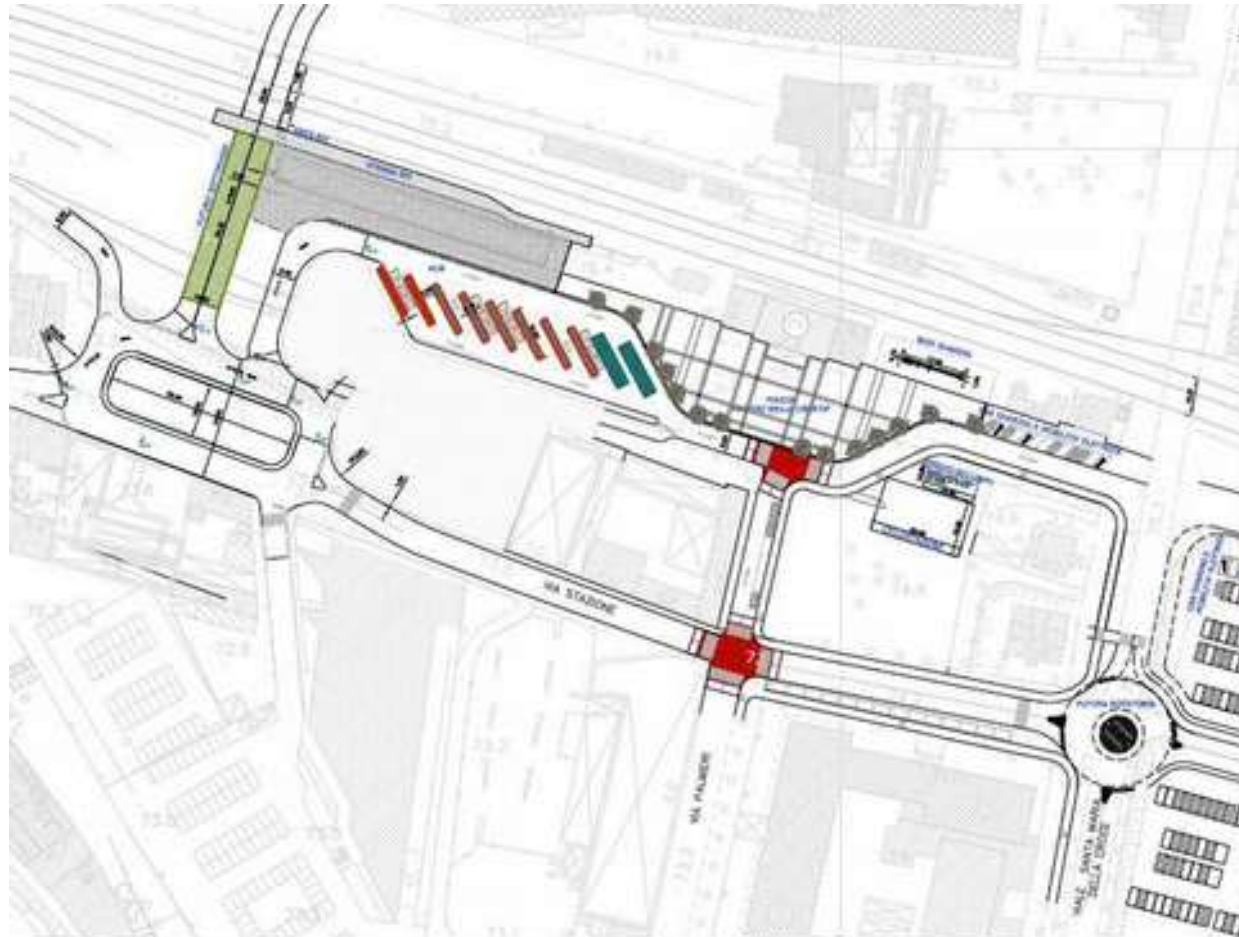
PLANIMETRIA GENERALE
